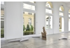
Misfits Y , 2021
